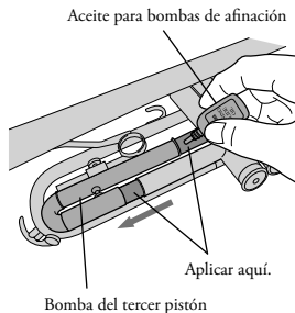
Bomba del tercer pistón
